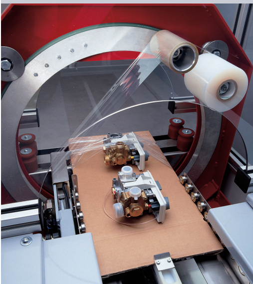
Automatische Fixierung durch Umwickeln.
